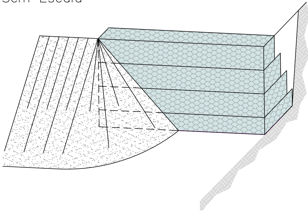
Detalhe do Fechamento Lateral Sem Escala
