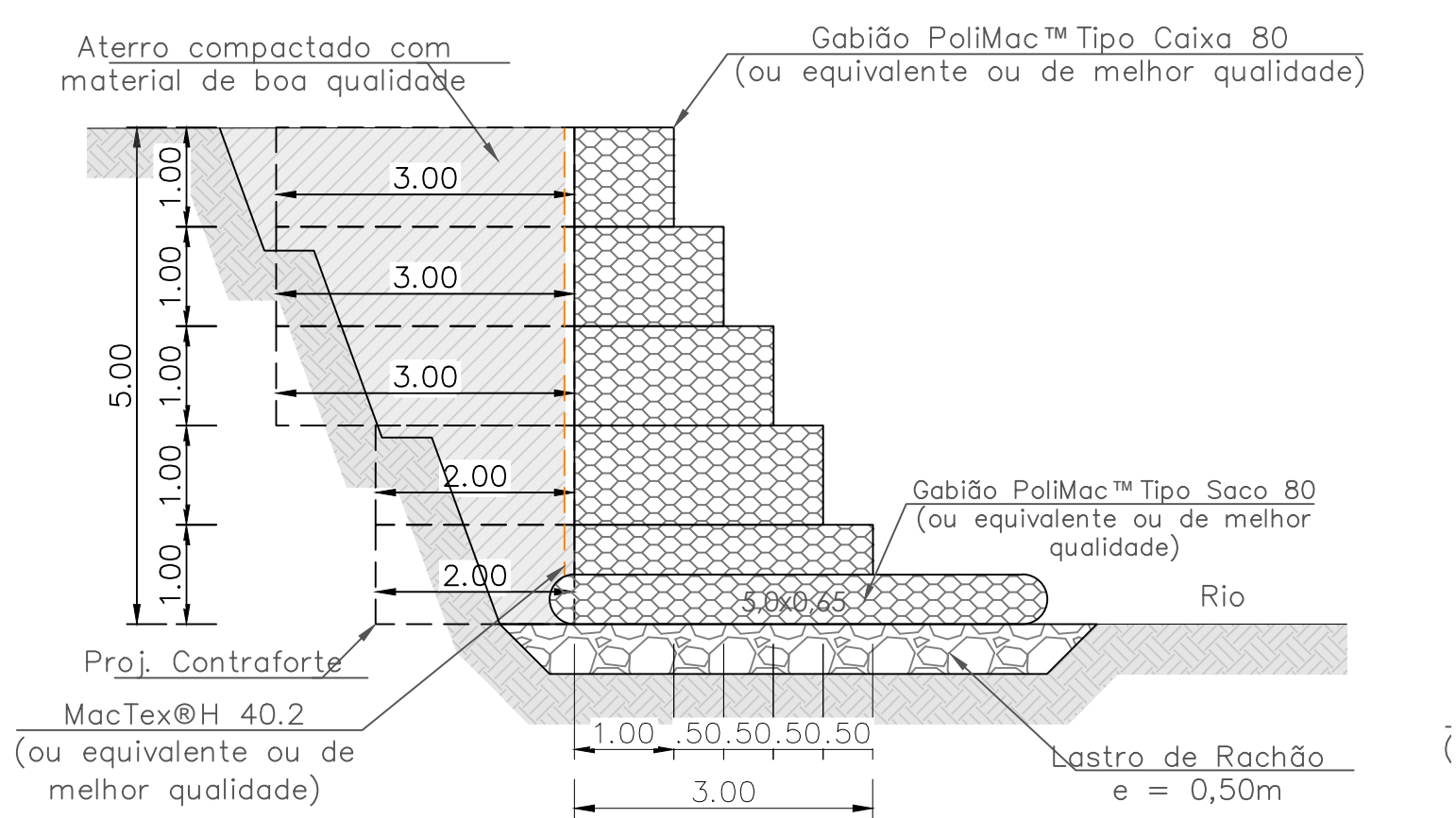
Planta Esquemática | Sem escala
