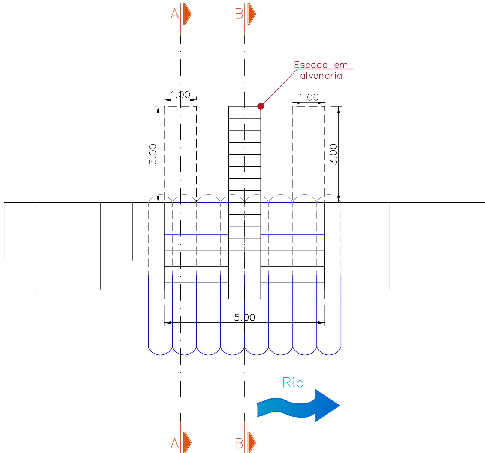
Planta Esquemática | Sem escala
