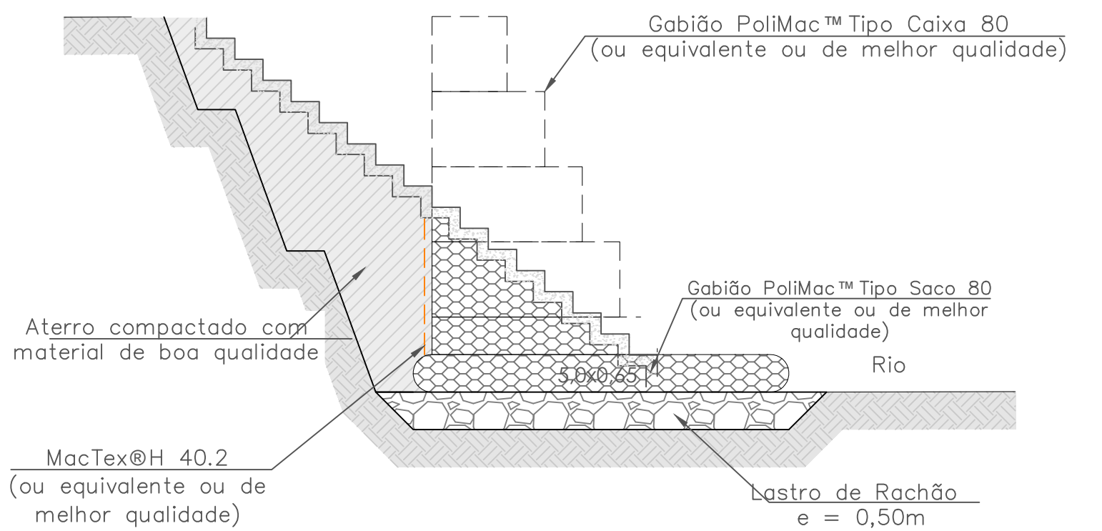
Planta Esquemática | Sem escala
